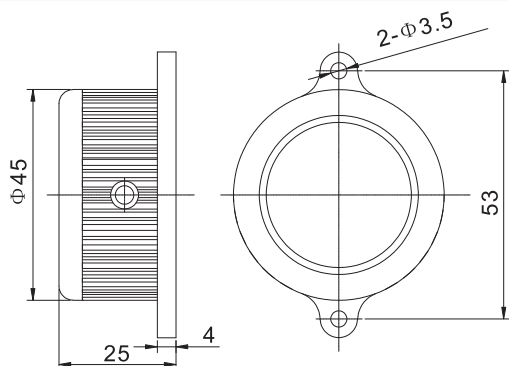
2 Montagelöcher D=3,5mm, Abstand 53mm
