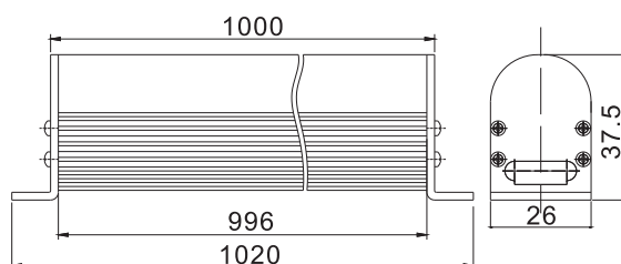
2 Montagelöcher D=4.0mm
