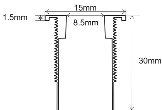
Écrou M12x1 / surplat 14mm O-Ring 1mm
